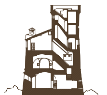
Sezione trasversale.
