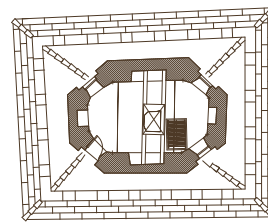
Pianta a quota +25.94
